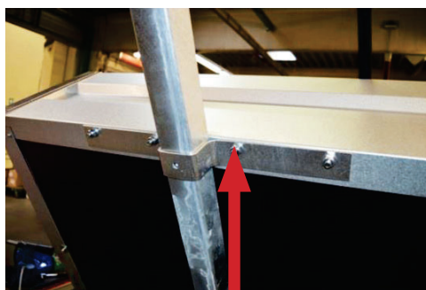
massive Deichselhalterung
