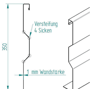
Wandprofil leichte Ausführung
